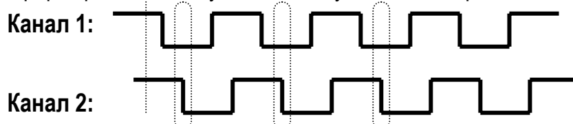
Рисунок 2 – Диаграмма формирования импульсов по входным каналам ДИ-О-5.
