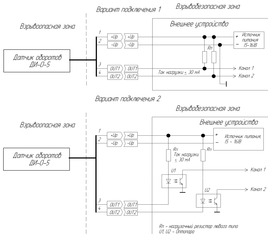
Рисунок А.4 - Схема электрическая подключения ДИ-О-5.3, ДИ-О-5.5
